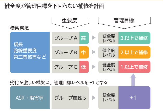
図A 橋梁のグループ化と管理レベル
